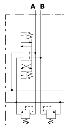
Esempio tipo P
