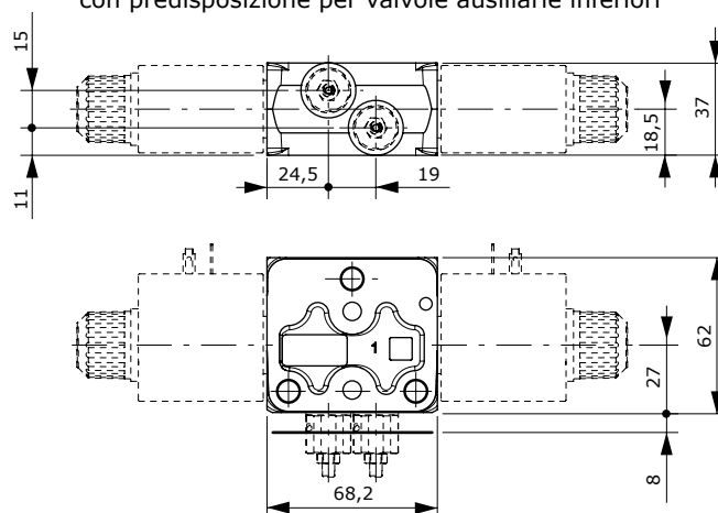
Esempio tipo Q
