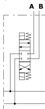
Esempio tipo Q
