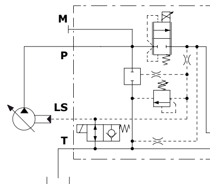
Esempio tipo AN16 per circuito a Centro Chiuso
