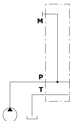
Tipo AN-ANB Bocche P e T aperte
