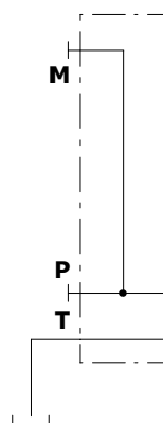
Tipo ANT-ANTB Bocca P tappata e T aperta
