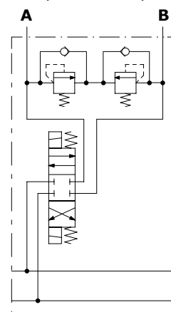
Esempio tipo PFL
