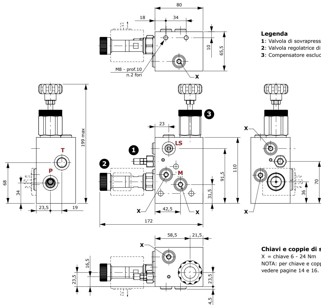
Esempio tipo AN6 per circuito a Centro Aperto
