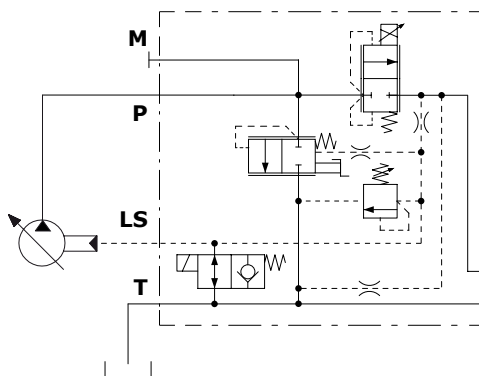
Esempio tipo AN15 per circuito a Centro Aperto e Chiuso
