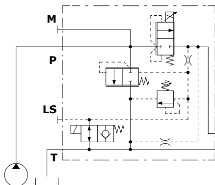
Esempio tipo AN14 per circuito a Centro Aperto
