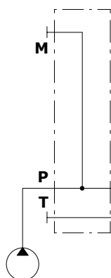
Tipo ANP-ANPB Bocca P aperta e T tappata
