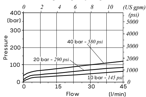
Setting range spring nr.1
