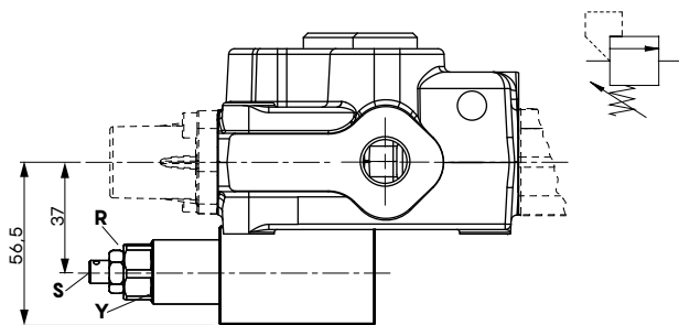
VSB valve
