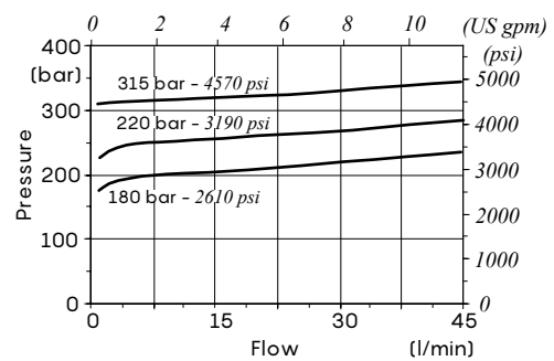
Setting range spring nr.4
