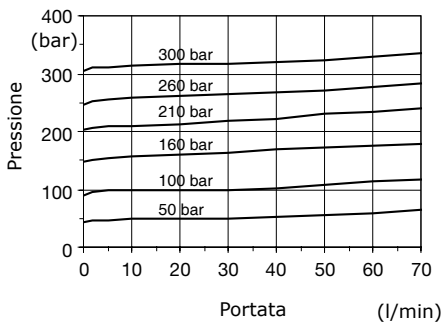
Valvole a taratura fissa tipo U Esempi di taratura (10 l/min)
